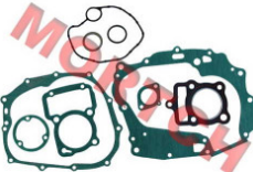
CG150 全车垫片 MICG150-1095
