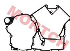
曲轴箱垫片 MICF0JWA-011001-30000
